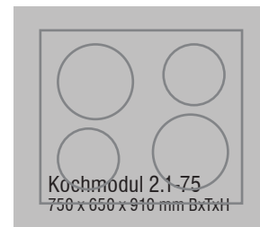
Kochmodul 2.1-75 750 x 650 x 910 mm BxTxH
